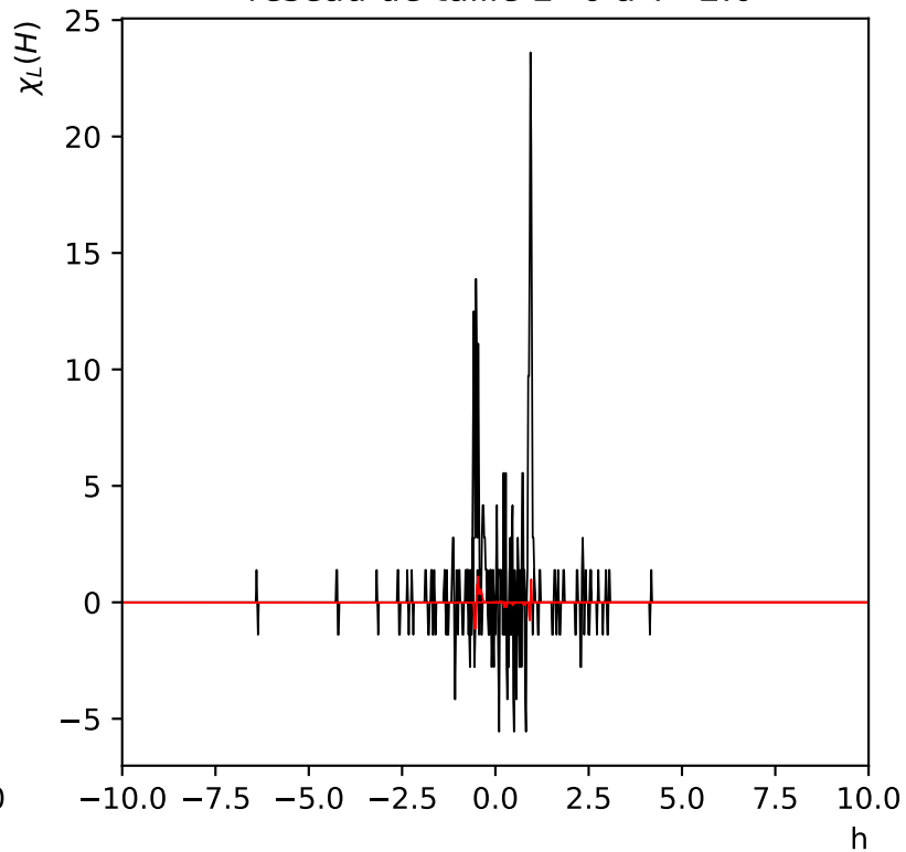
\chi_L(H) réseau de taille L=6 à T=2.0
