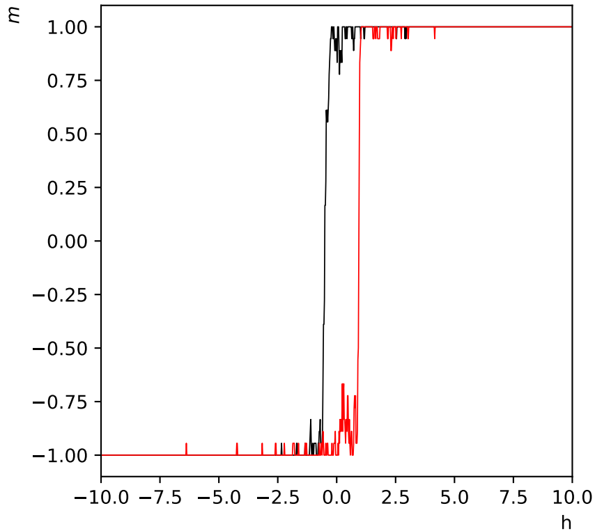
Hystérésis de l'aimantation réseau de taille L=6 - h=10 à T=2.0
